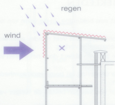
Figuur 4.5.2 Voorbeeld van kapafdichting
