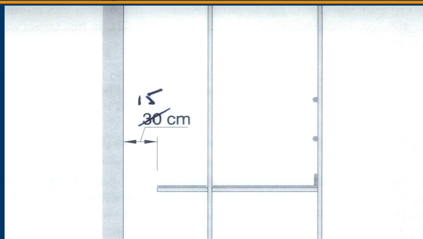
Figuur 4.7 Maximale afstand tussen steigervloer en object/gevel
